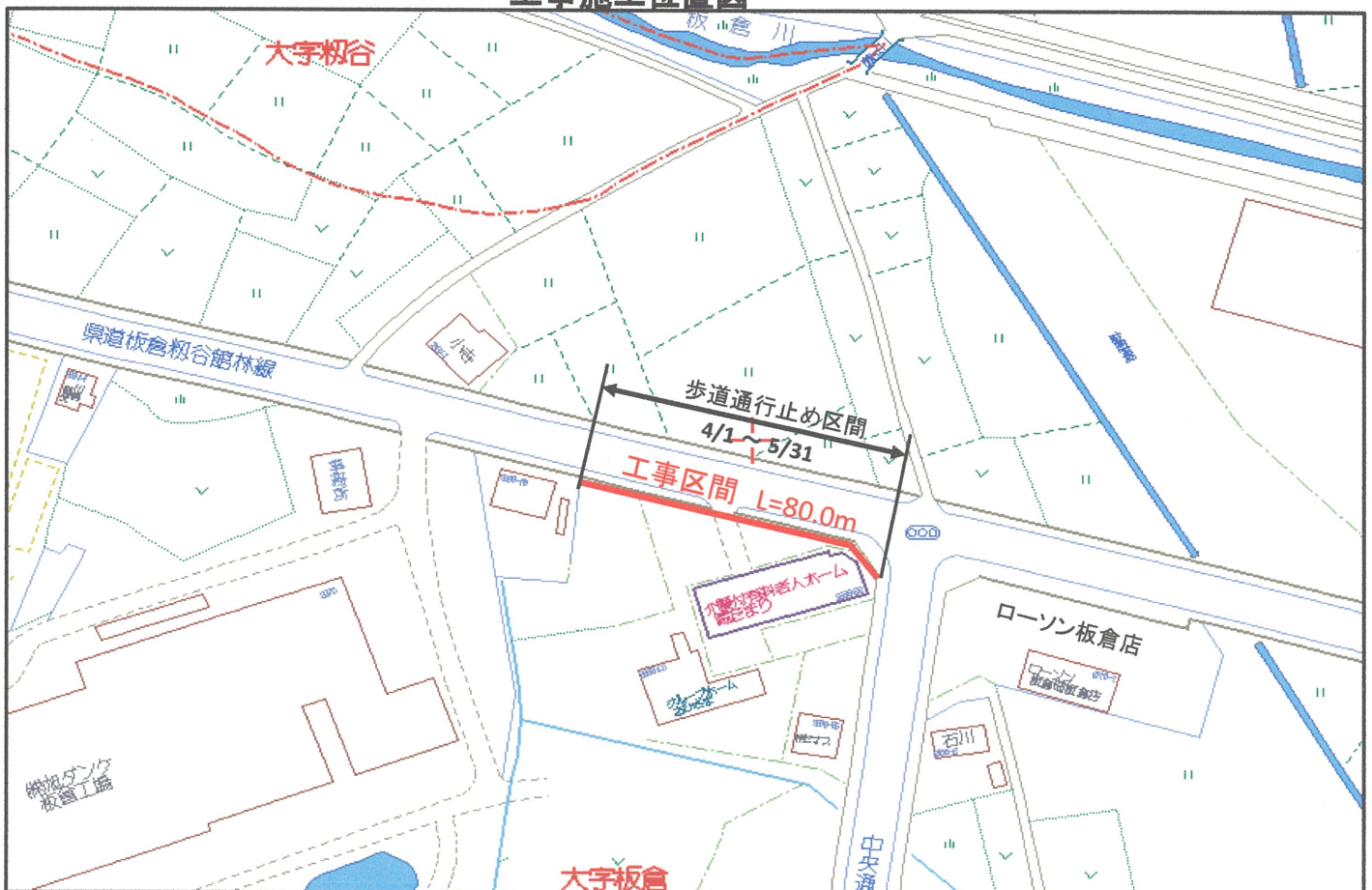
工事施工位置図
